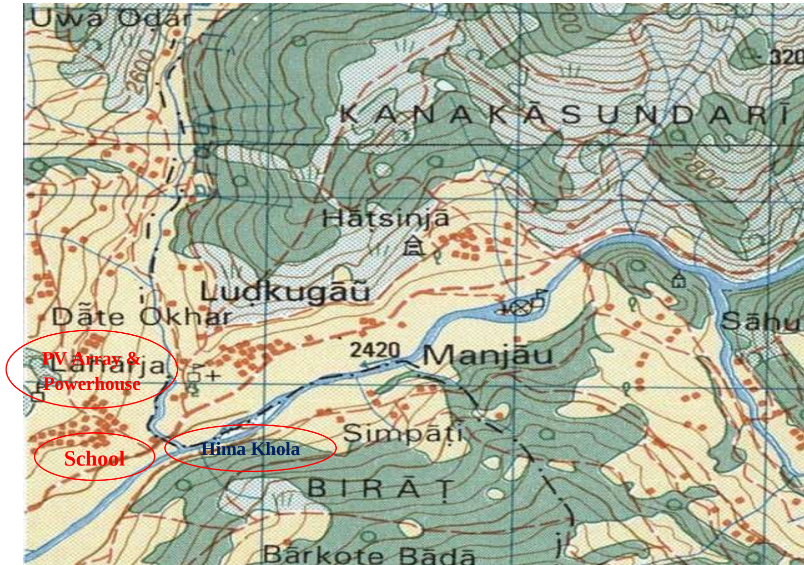
Figure 2: Topographic Map of Kankasundari Solar Mini Grid Subproject
